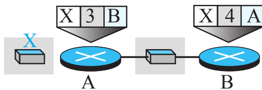
(d) Después de B es actualizado por A
