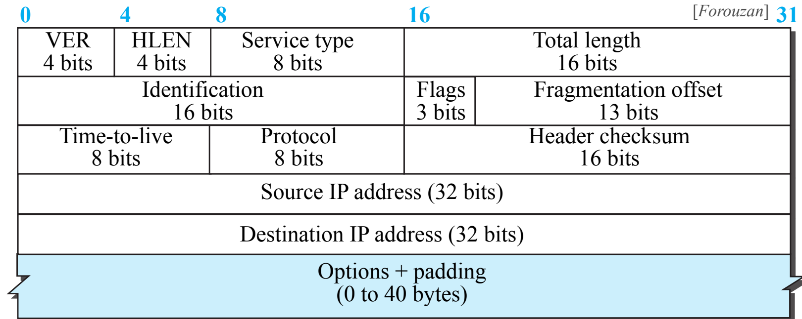
(b) Cabecera IP
