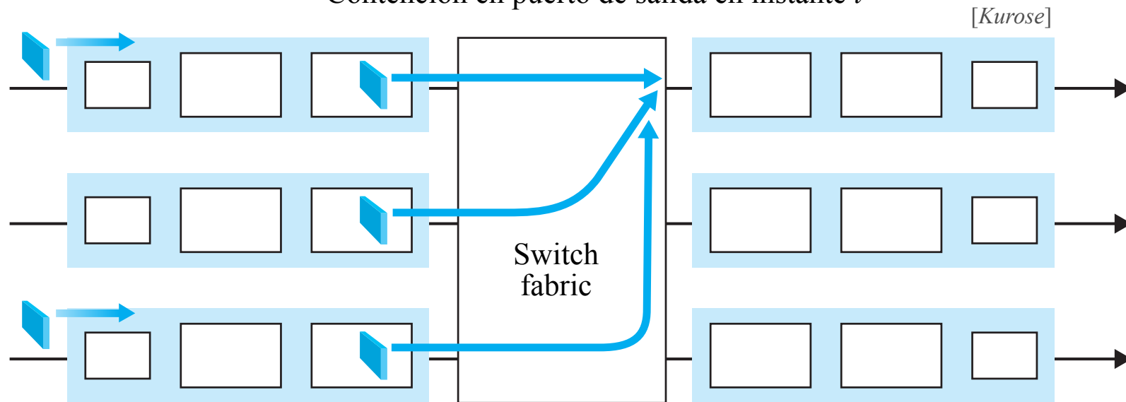
Contención en puerto de salida en instante t
