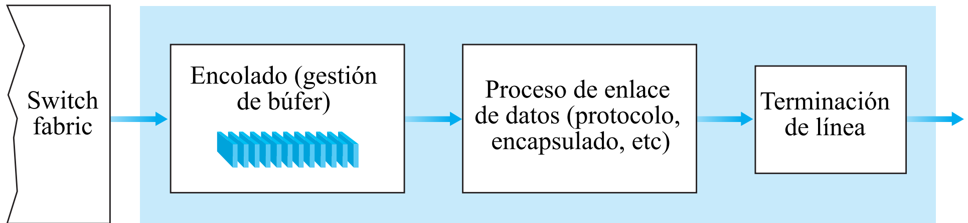
(b) Procesamiento en puerto de salida
